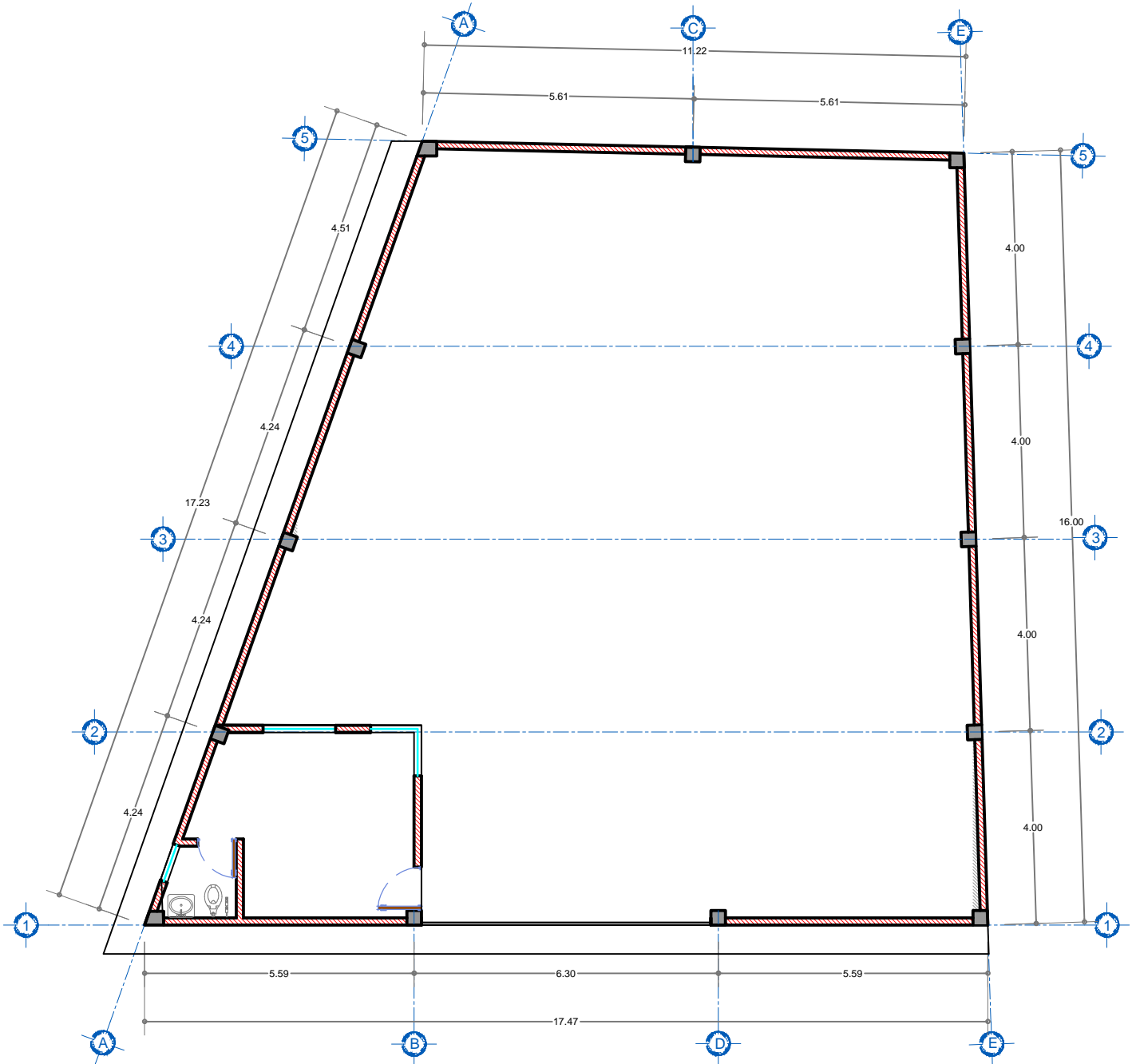
PLANTA ARQUITECTÓNICA Escala 1-1/25 Acotación: Metros SUP. DE CONSTRUCCION = 60.74 M2
